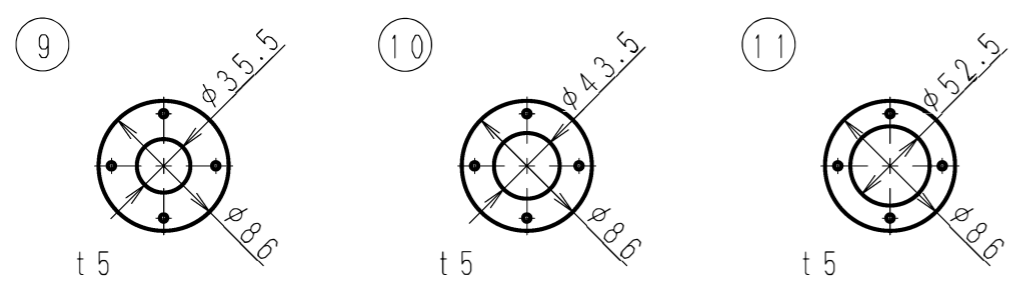
付属品 詳細図 (SCALE 1:5)
