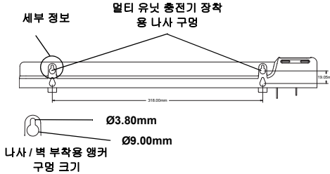
그림 3: 벽면 장착 가능
