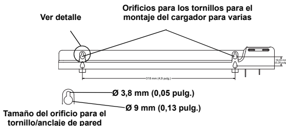
Figure 3: Características del montaje en pared
