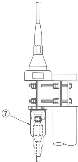
●取付状態図
