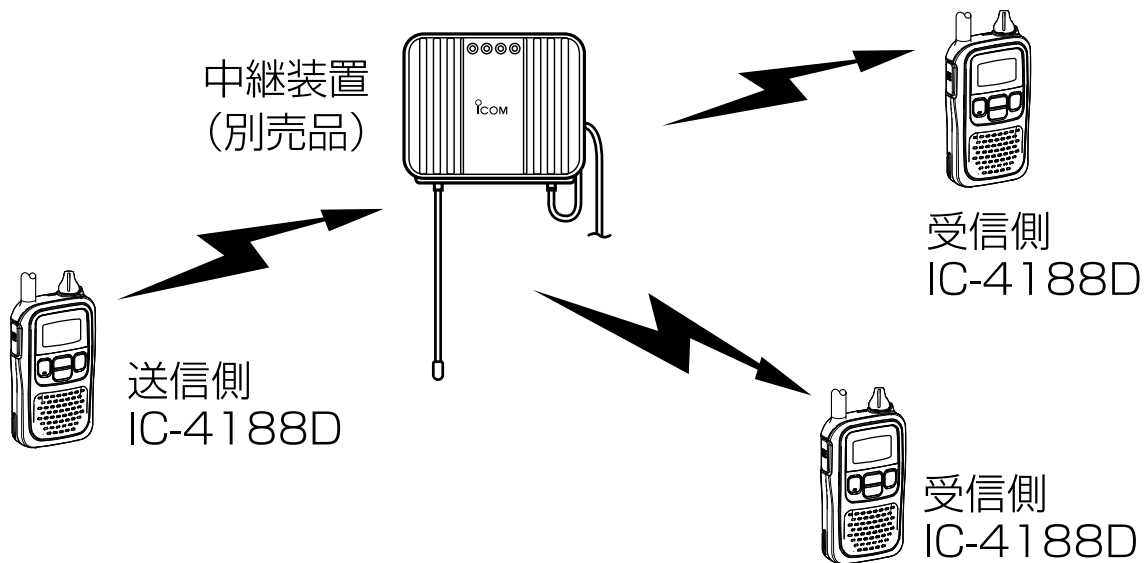
中継システム構成図
